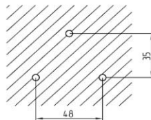
Bohrbild
