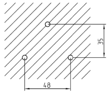
Bohrbild
